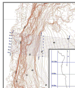
等高線平面図 と横断箇所
